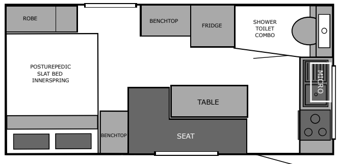
15'X7'6"-2 SPRINTER
