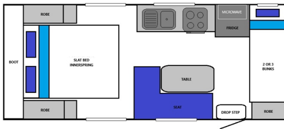
MARATHON 18' - 1
