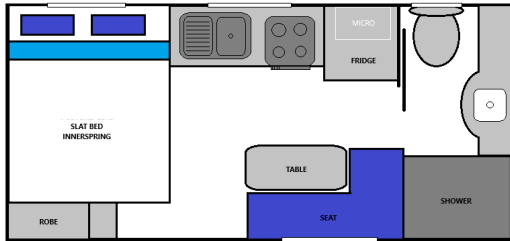
MARATHON 15'6" - 1
