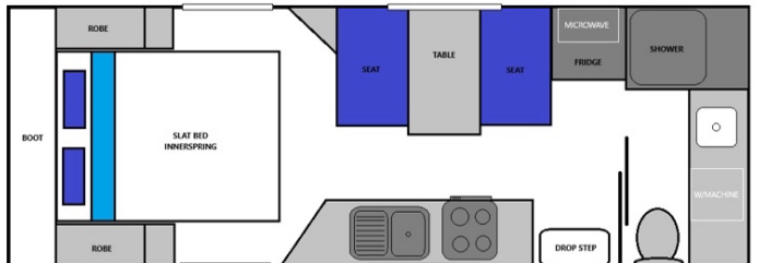
MARATHON 19'6" - 3
